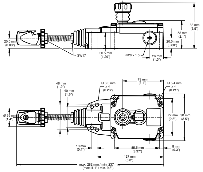
RP-RM83F-..LT..
