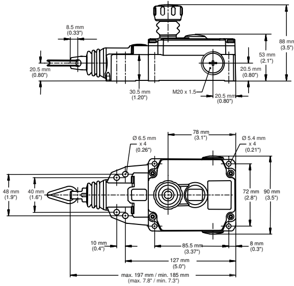
RP-RM83F-..LR..
