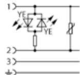
11.024-K, 3-pin + PE
