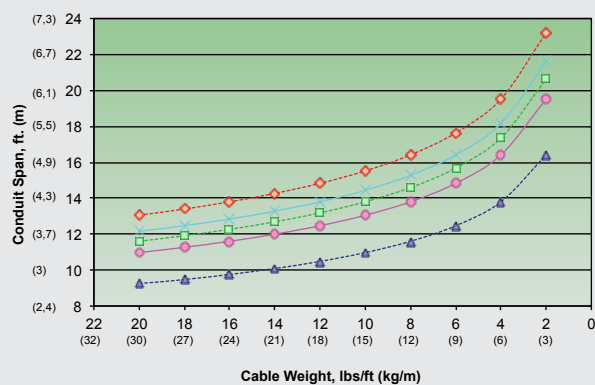
4 1/2" (116 mm) HW Conduit (ID only)
