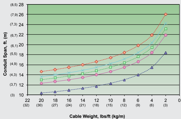
6" (155 mm) SW Conduit (IPS & ID)
